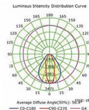
30W QKSMS-TGD-1132 50W QKSMS-TGD-1133 70W QKSMS-TGD-1134 100W QKSMS-TGD-1135
