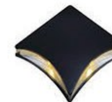
Model: QKSM-BD1705 Watt: 4*1W Material: Aluminum die casting Size: 205*206*73mm
